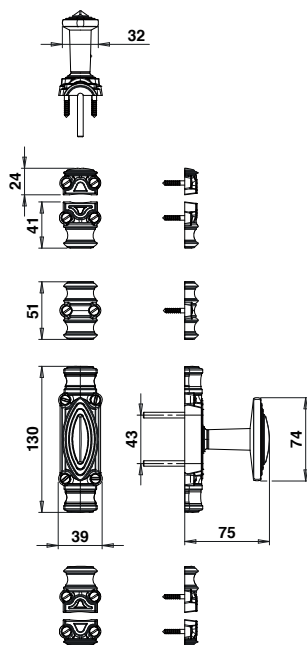
136MEA.. Fausse crémonne légère n°136 - Fonte Bouton rustique médium
