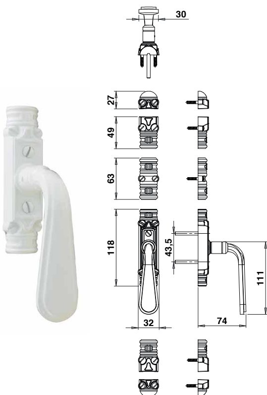
138RBB.. Fausse crémonne étroite n°138R - Zamak Béquille bec de canard
