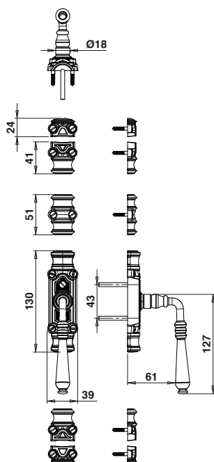
136BCA.. Fausse crémonne légère n°136 - Fonte Béquille coudée
